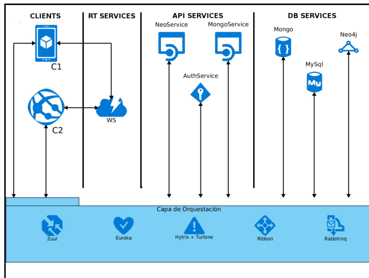
Figura 7: Arquitectura final de Whaya.
