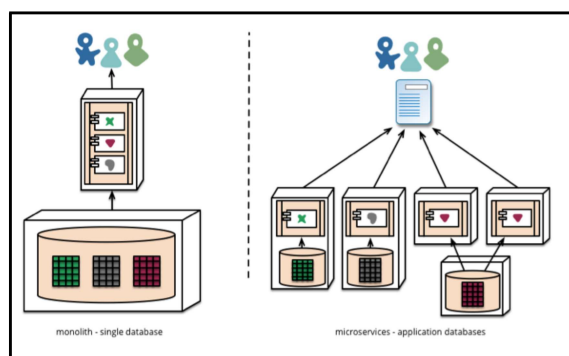
Figura 3: Arquitecturas monolíticas vs microservicios. [2]
