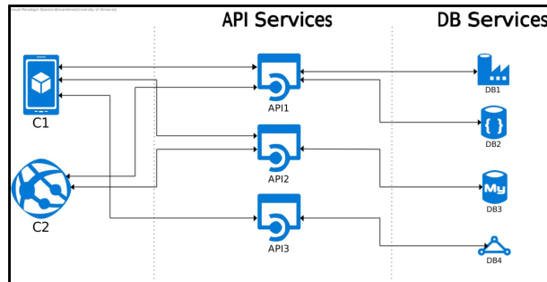
Figura 5: Arquitectura básica objetivo Whaya.
