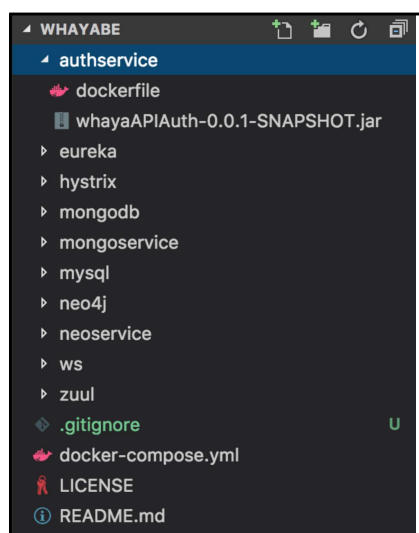
Figura 4: Scaffolding de WhayaBe.
