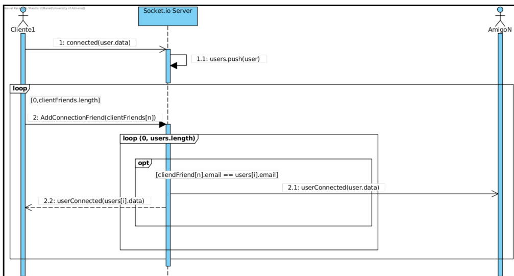
Figura 13: Diagrama de secuencia WS.
