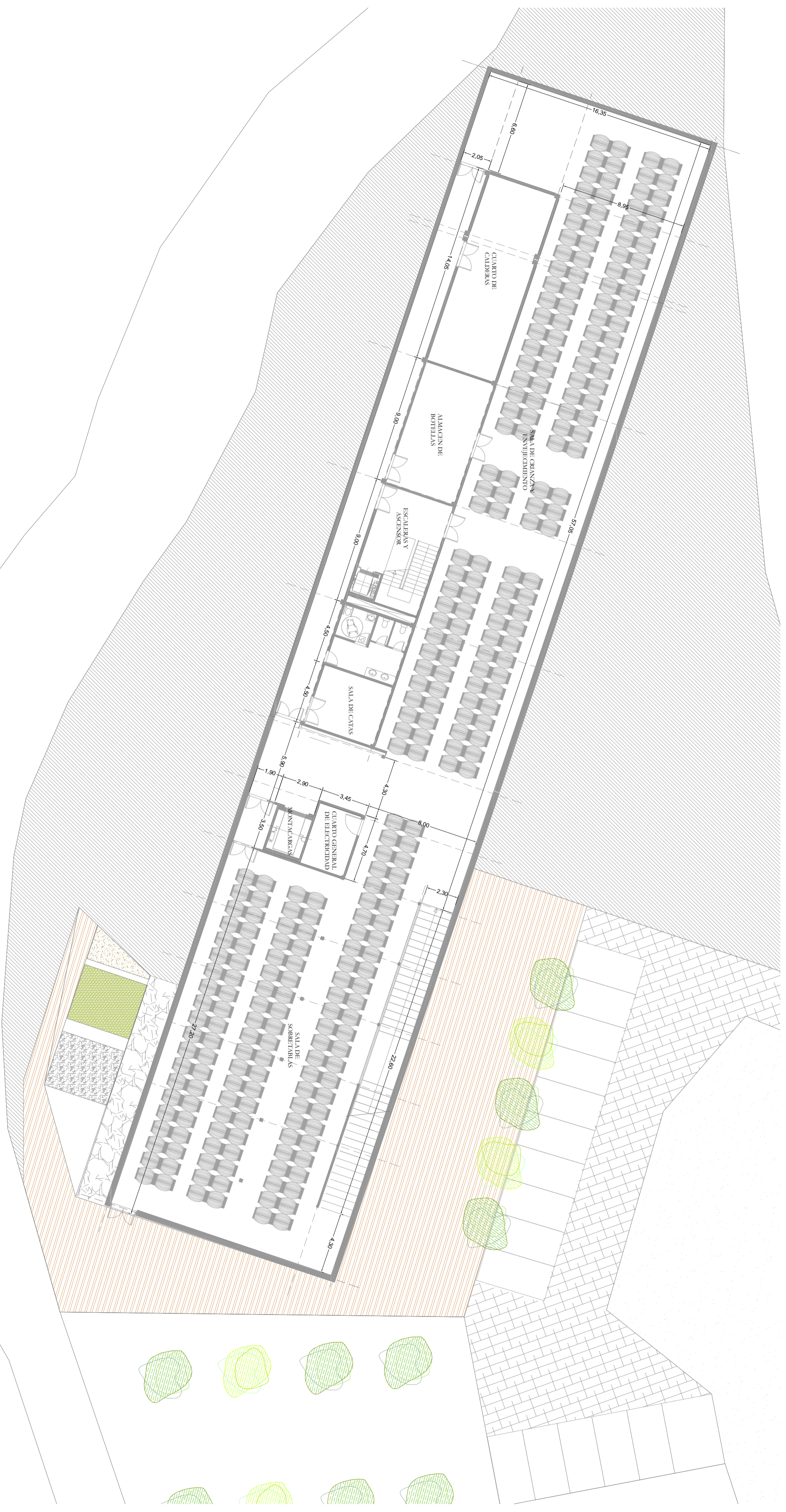
PLANTA SÓTANO (-9 m)
