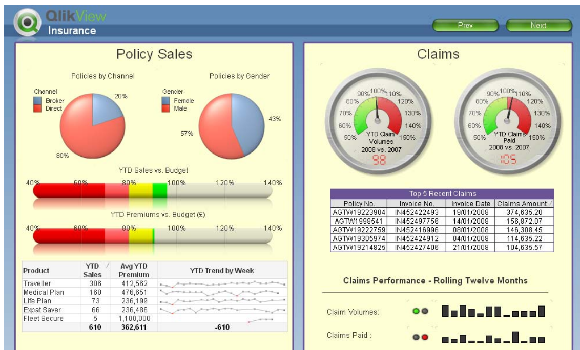
Figura 38. CMI QlikView.
