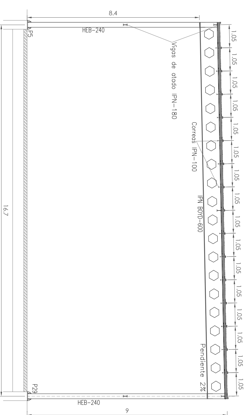
Pv5. Sección A-A' Módulo de producción e 1:100
